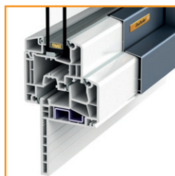
Sanierungs-Blendrahmen
